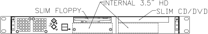
Front in-side (Disk Option 2)
